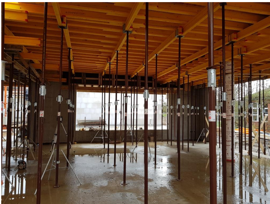
Bild Nr.: 5 | Datum: 11.03.2020 | Deckenschalung und Schalungstützen für die Decke über EG
