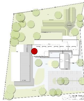
Bild Nr.: 4 | Datum: 17.06.2019 | Gebäudetrennung als vorbereitende Maßnahme für die Abbrucharbeiten
